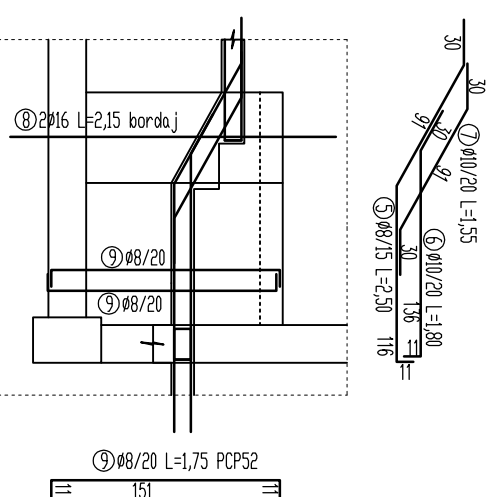
DETALIU ARMARE TREPTÉ INTRARE BUCATARIE
