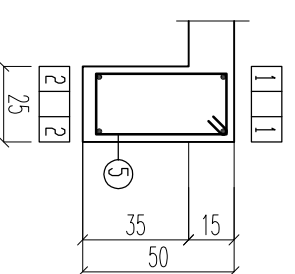
SECȚIUNEA 1-1 (1:25)
